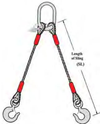
2 Leg Redi-Grip® Sling
