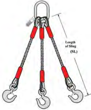
3 Leg Redi-Grip® Sling
